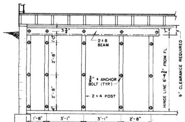
SECTION A-2
